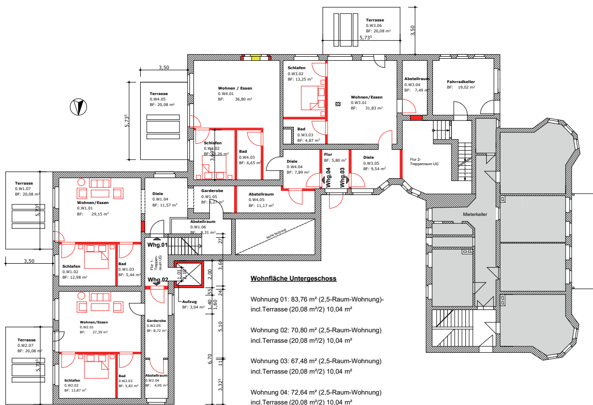
Untergeschoss
